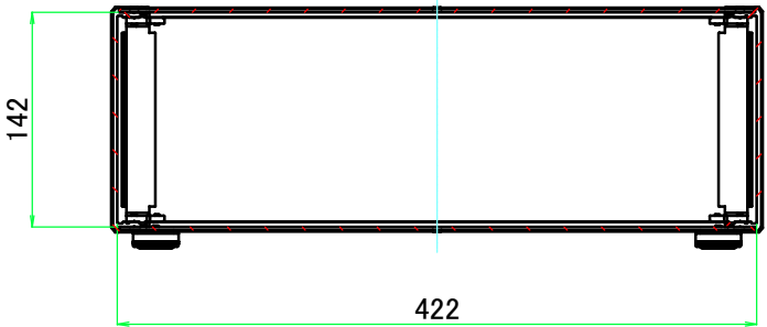
A-A ( 1 : 5.5 )
