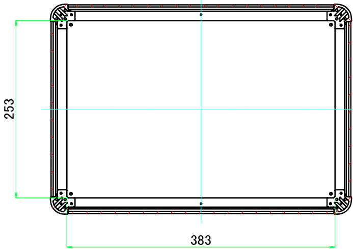
C-C ( 1 : 5.5 )
